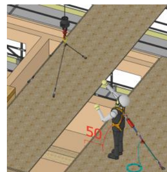
Oder Sicherung mit PSAgA an Absturzkanten bei Elementverlegung
